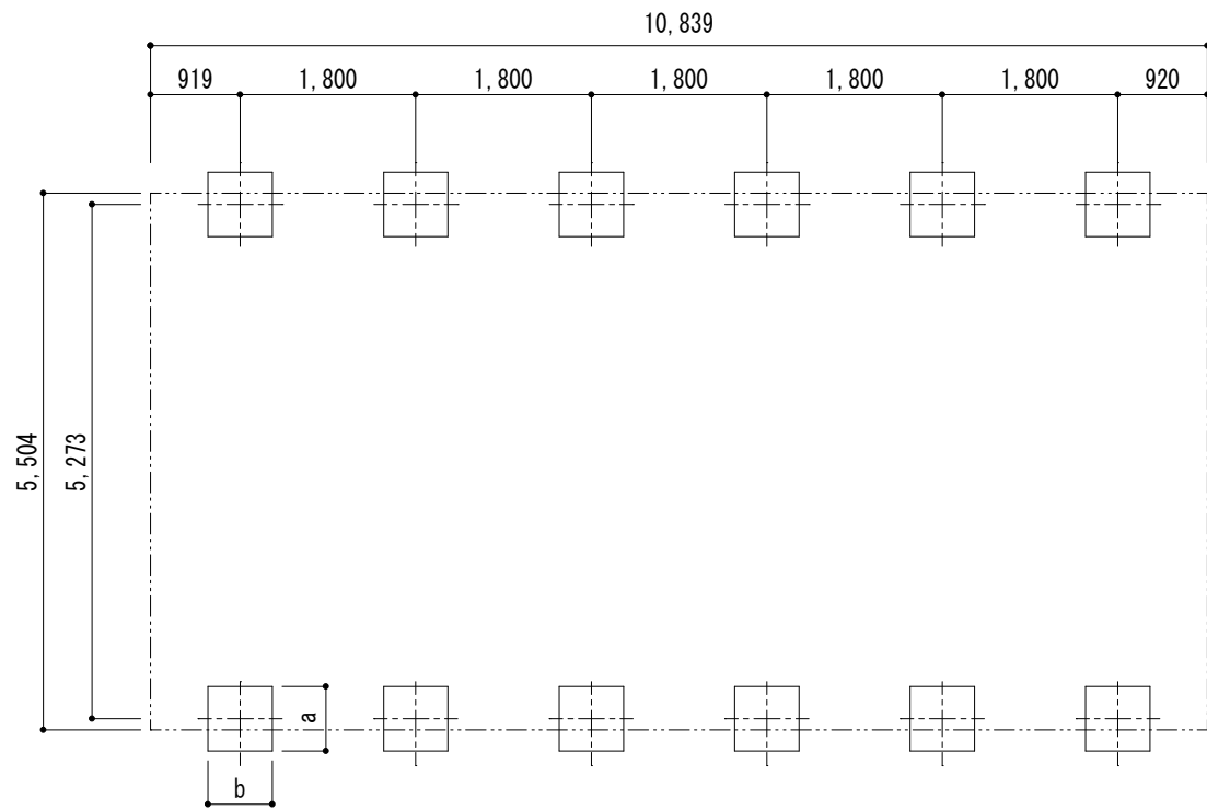
■基礎配置図
